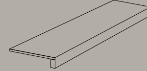
SCALINO INCOLLATO GLUED STEP TREAD / NEZ DE MARCHÉ COLLÉ / GEKLEBTE STUFENPLATTE / PELDAÑO CON PERFIL PEGADO 33x120 (13"x48") RT 9 mm
