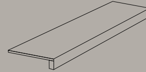
SCALINO CON PROFILO INCOLLATO GLUED STEP TREAD / NEZ DE MARCHÉ COLLÉ / GEKLEBTE STUFENPLATTE / PELDAÑO CON PERFIL PEGADO 30x120 (12"x48") RT 9 mm
