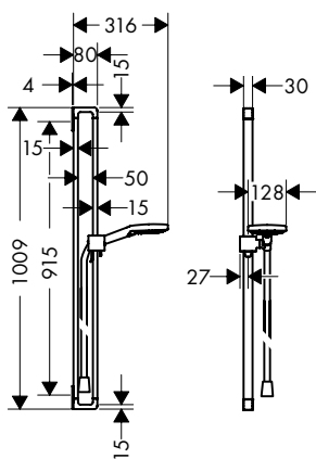
Душевой набор, 0,90 м, с ручным душем 120 Jet
