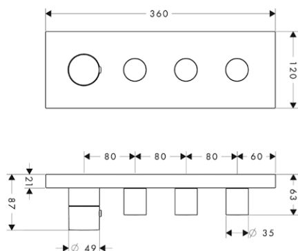
Модуль термостата, 360/120, для 3 потребителей, скрытого монтажа
