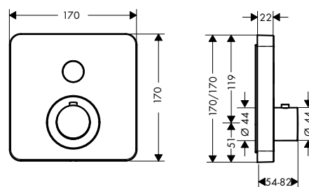
Термостат для 1 потребителя, скрытого монтажа, softcube
