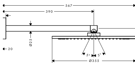
Верхний душ 350 Jet, с держателем
