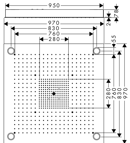
ShowerHeaven 970/970 3jet, с подсветкой
