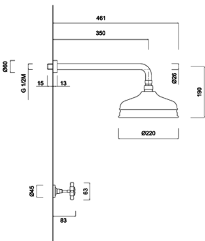
ART. 3715W2 RUBINETTI INCASSO PER DOCCIA E DEVIATORE 2 VIE CONCEALED SHOWER TAPS AND 2 WAYS DIVERTER
