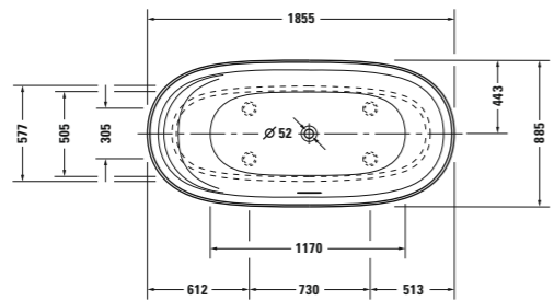
# 700330 00 00 0000, 1855 x 885 mm Freistehend. Freestanding. Exenta
