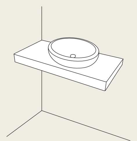
installazione da appoggio su piano on top installation 60 x 45 x h14,5 - FLLA60
