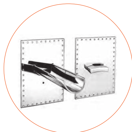
Cod. 55538/22 Gruppo lavabo a parete composto da bocca incasso mm. 220 e miscelatore su piastre separate con scatole incasso, collegamenti interni, dispositivo di regolazione portata acqua, cartuccia progressiva. Wall basin mixer with 220 mms. spout and mixer on separate plates with built-in boxes, internal connections, flow regulations system, progressive cartridge
