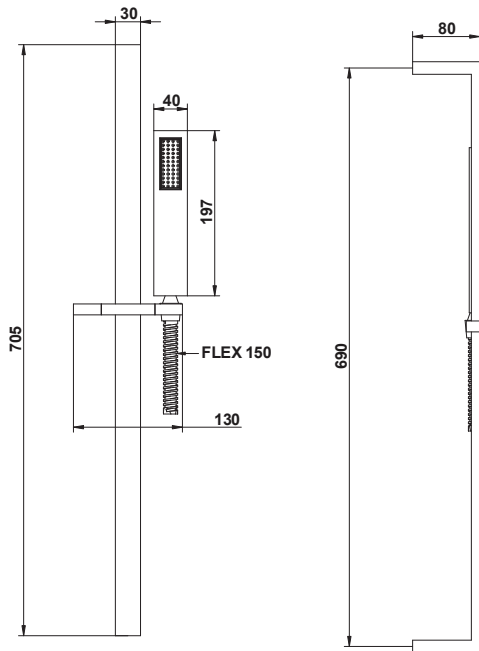
Cod. 878 Saliscendi rettangolare con doccetta monogetto e flessibile doppia aggraffatura mm 1500, 1/2" ff conico. Rectangular minimalist sliding rail with single function handshower and mms 1500 double interlock hose, 1/2" ff conical.
