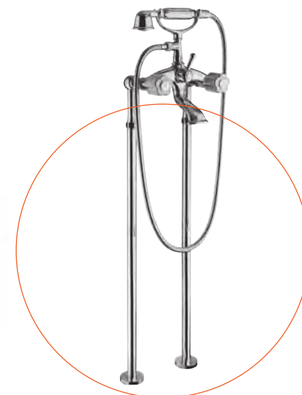
Cod. 11528 Blanc / White Cod. 12528 Noir / Black Gruppo vasca esterno su colonnette da terra con set doccia External bath and shower mixer to the floor with shower set
