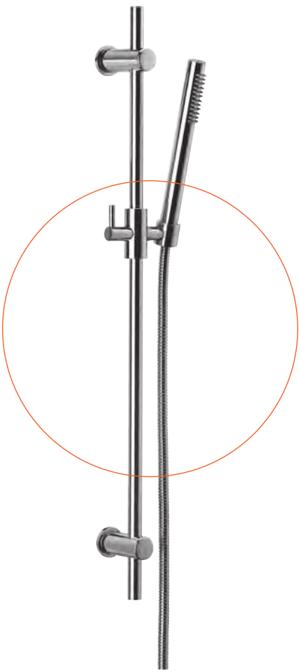
Cod. 870 Saliscendi minimalista tondo con doccetta monogetto e flessibile doppia aggraffatura mm 1500, 1/2" ff conico. Round minimalist sliding rail with single function handshower and mms 1500 double interlock hose, 1/2" ff conical.
