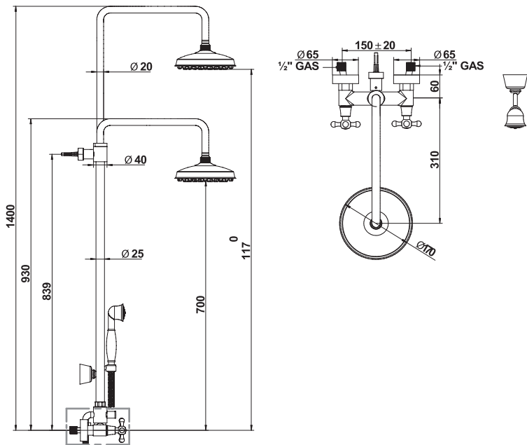
DETTAGLIO A / DETAIL A Regolatore da 6 l/min. e valvola di non ritorno 6 l/m limitation system and not return valve
