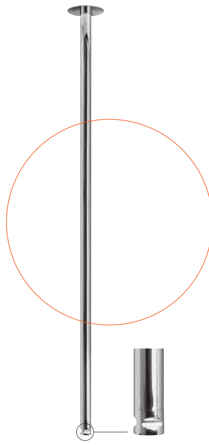
Cod. 977/M Bocca da soffitto con miscelatore incorporato e cartuccia progressiva. Spout from ceiling with mixer included in the spout and progressive cartridge.
