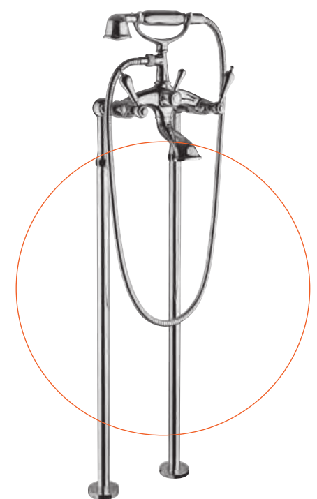
Cod. 17528 Gruppo vasca esterno su colonnette da terra con set doccia External bath and shower mixer to the floor with shower set
