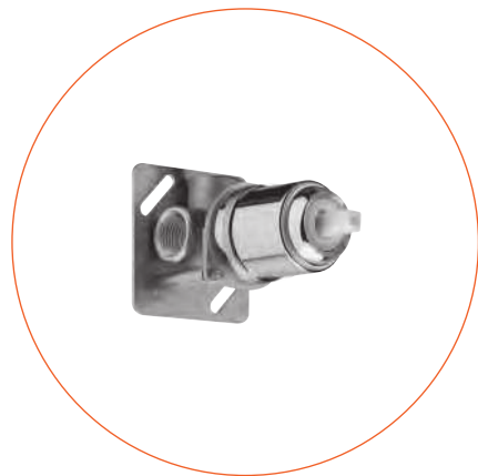
Cod. 9730/M Corpo miscelatore incasso Ø 35 mm. con flangia per installazione su muro solido Ø 35 mms. built-in mixer with built-in flange for concrete wall
