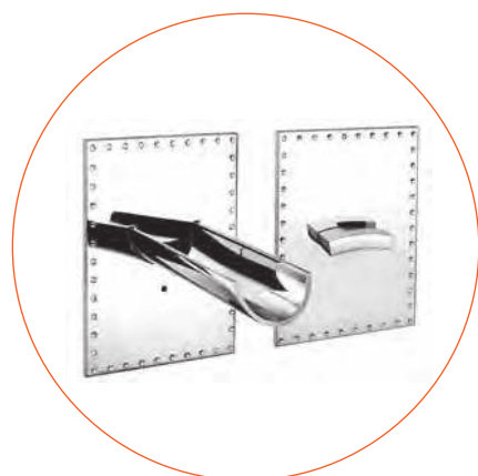
Cod. 55538/12 Gruppo lavabo a parete composto da bocca incasso mm. 120 e miscelatore su piastre separate con scatole incasso, collegamenti interni, dispositivo di regolazione portata acqua, cartuccia progressiva. Wall basin mixer with 120 mms. spout and mixer on separate plates with built-in boxes, internal connections, flow regulations system, progressive cartridge.
