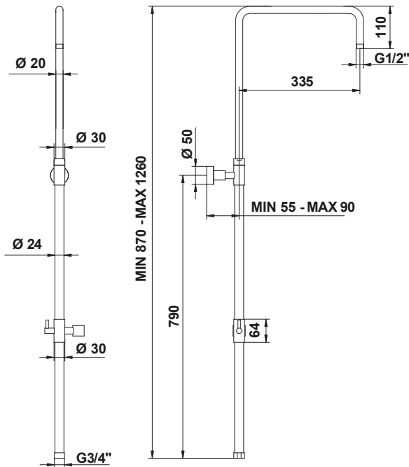
Cod. 813 Tubo doccia orientabile senza deviatore con supporto doccia scorrevole su tubo. Orientable shower tube without diverter, with shower sliding support.
