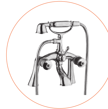
Cod. 06527 Trasparente / Transparent Cod. 65527 Blu e rosso / Blue and Red Gruppo vasca esterno su colonnette con set doccia External bath and shower mixer on pillar connection with shower set
