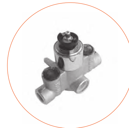
Cod. 9700 Corpo miscelatore termostatico incasso. Built-in thermostatic mixer. per/for cod. 40554
