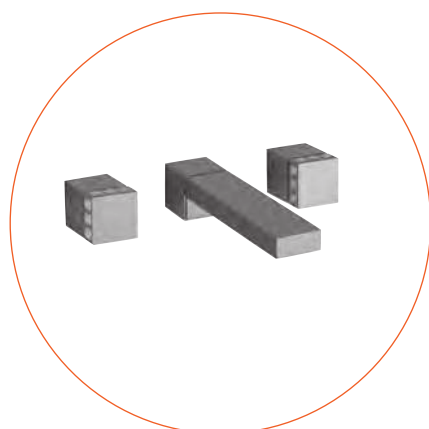
Cod. 6P538/22Z OPEN BOX Gruppo lavabo incasso 3 fori con bocca 220 mm Predisposto per fissaggio su OPEN BOX 3-holes built-in basin mixer with 220 mms. spout With fixing connection for OPEN BOX
