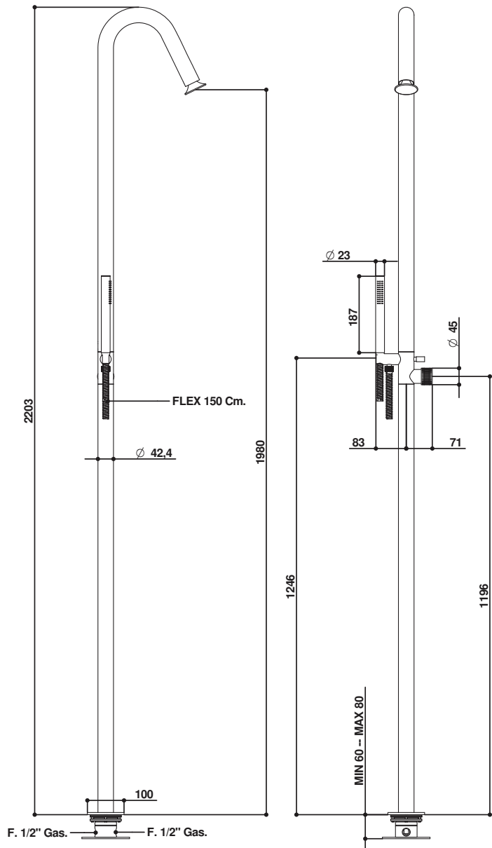
Corpo incasso Built-in body
