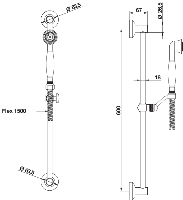
Cod. 871 - Cod. 971 Saliscendi classico con doccetta monogetto e flessibile doppia aggraffatura 1500 mm, 1/2" ff conico. Classic sliding rail with single function handshower and 1500 mms double interlock hose, 1/2" ff conical.
