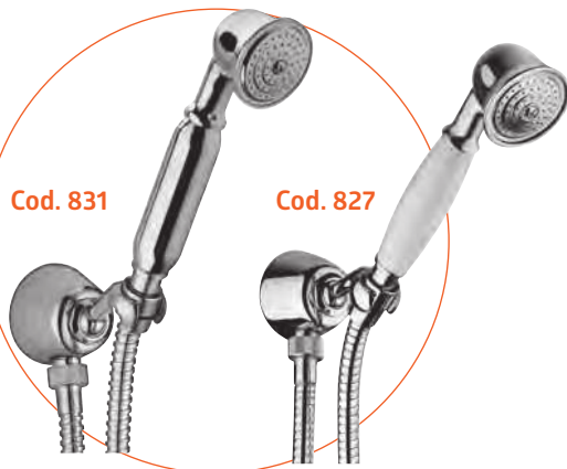
Cod. 831 - Cod. 827 Duplex con erogazione con supporto orientabile, doccetta monogetto e flessibile doppia aggraffatura 1500 mm, 1/2" ff conico. Shower set with water supply elbow with orientable bracket, single function handshower and 1500 mms double interlock hose, 1/2" ff conical.
