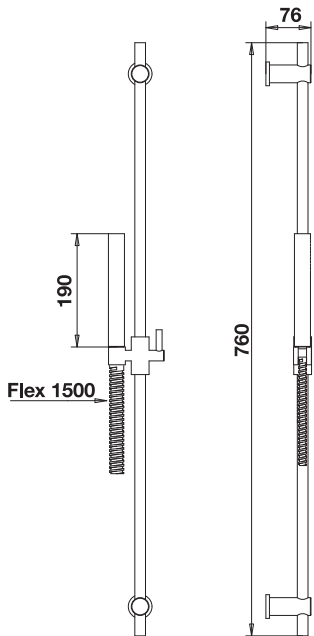
Cod. 870 Saliscendi minimalista tondo con doccetta monogetto e flessibile doppia aggraffatura mm 1500, 1/2" ff conico. Round minimalist sliding rail with single function handshower and mms 1500 double interlock hose, 1/2" ff conical.
