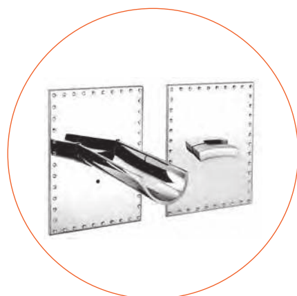
Cod. 55538/18 Gruppo lavabo a parete composto da bocca incasso mm. 180 e miscelatore su piastre separate con scatole incasso, collegamenti interni, dispositivo di regolazione portata acqua, cartuccia progressiva. Wall basin mixer with 180 mms. spout and mixer on separate plates with built-in boxes, internal connections, flow regulations system, progressive cartridge
