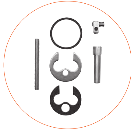
Cod. 9947 Set fissaggio / Set fix per/for cod. ..501 - 503 - 521 - 522 - 581 - T CROSS - T LEVER
