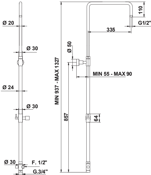
Cod. 814 Tubo doccia orientabile con deviatore e supporto doccia scorrevole su tubo. Orientable shower tube with diverter and shower sliding support.
