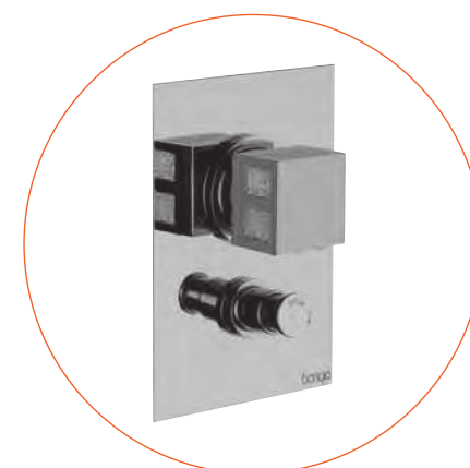
Cod. 3D529 Miscelatore incasso doccia con deviatore, cartuccia progressiva con scatola incasso BONGIO BOX Built-in shower mixer with diverter, progressive cartridge and BONGIO BOX built-in box
