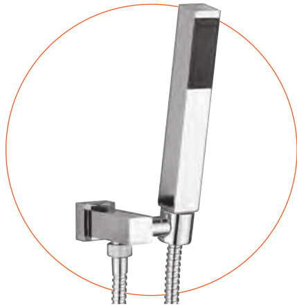
Cod. 834 Duplex minimalista quadro con erogazione, supporto orientabile, doccetta monogetto e flessibile doppia aggraffatura mm 1500, 1/2" ff conico. Square shower set with water supply elbow, orientable bracket, single function handshower and 1500 mms double interlock hose, 1/2" ff conical.
