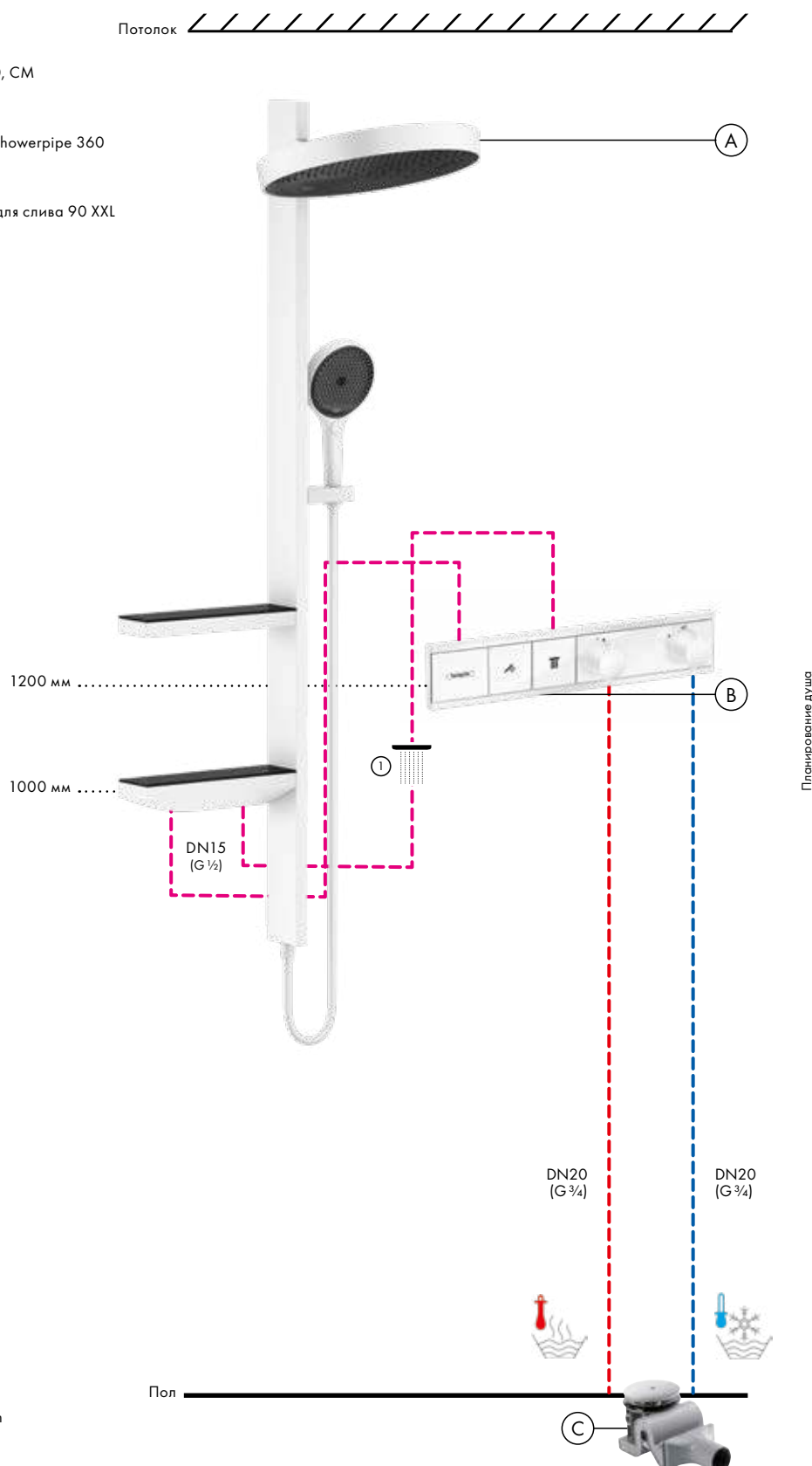
Скрытая часть Showerpipe 360 # 26840180
